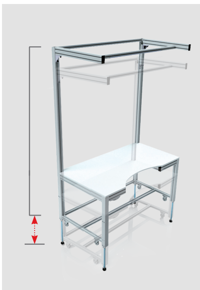
Synchroner Hub von Arbeitsfläche und Aufbauportal
