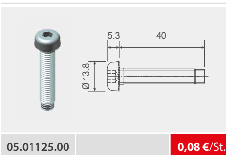
Flachkopfschraube SF 8 x 40, vz.
