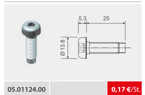
Flachkopfschraube SF 8 x 25, vz.
