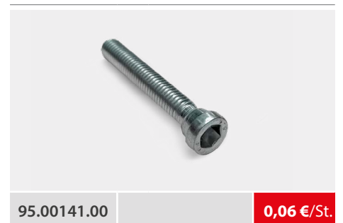
Kegelkopfschraube M6 x 45, vz.
