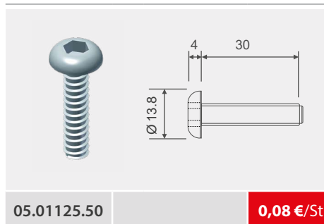
Flachkopfschraube SF 7,4 x 30-Ku, vz.
