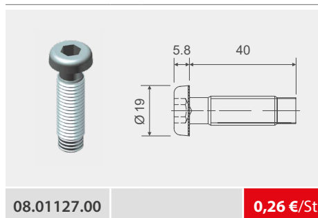
Flachkopfschraube SF 12 x 40, vz.
