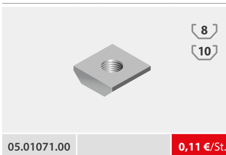
Nutenstein, flach • 8/10 | M6, vz.
