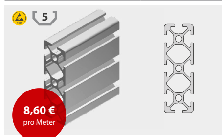
Aluprofil 20 x 60/Nut 5
