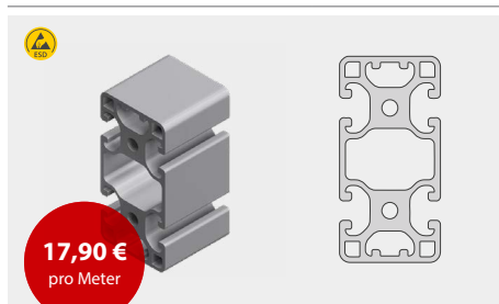
Aluprofil 40 x 80N-2N180
